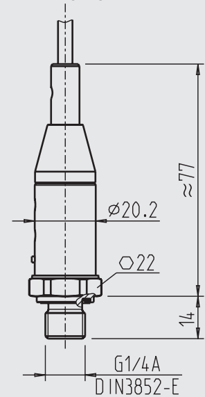
mit Kabelausgang
